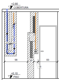
VISTA 1 - WC. ESC. 1 : 50
