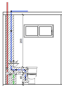
VISTA 3 - WC. ESC. 1 : 50
