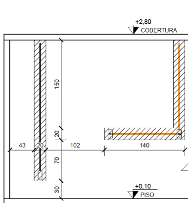
VISTA 2 - COZINHA ESC. 1 : 50
