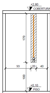
VISTA 2 - WC. ESC. 1 : 50
