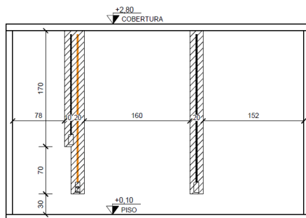
VISTA 2 - DORMITÓRIO 2
